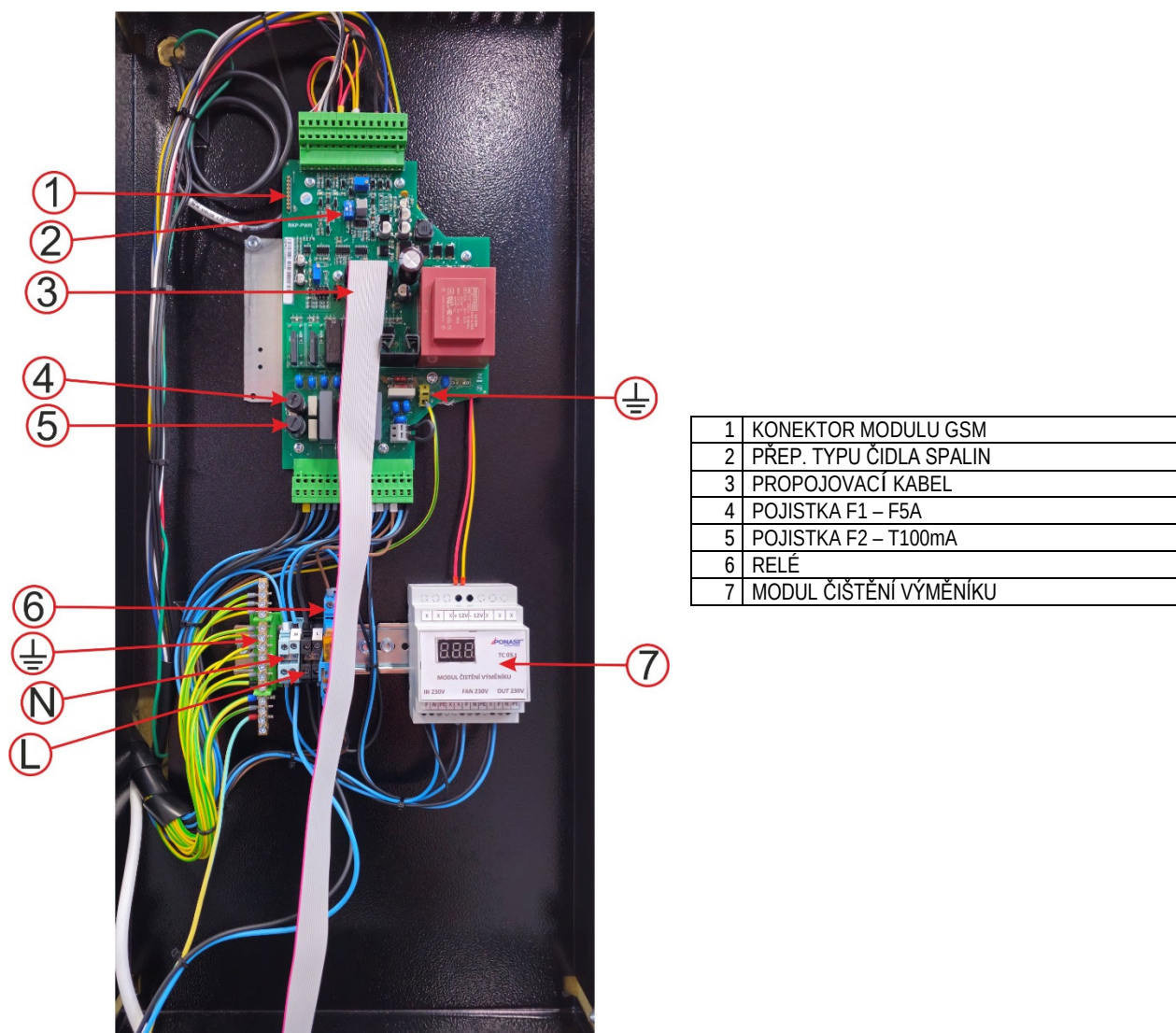
Obr. č. 2 Řídicí jednotka – zobrazení hlavních částí
