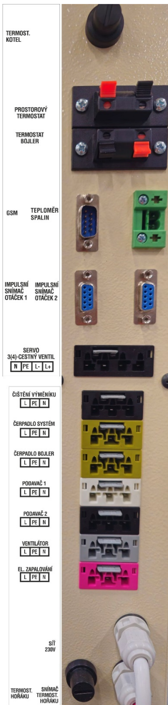
Obr. č. 4 Řídicí jednotka – přípojný panel s konektory
